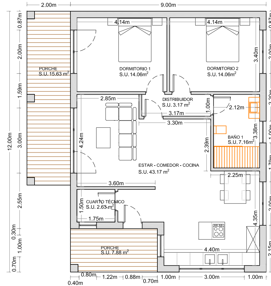
PLANTA BAJA SUP. CONSTRUIDA : 124,01 m 2
