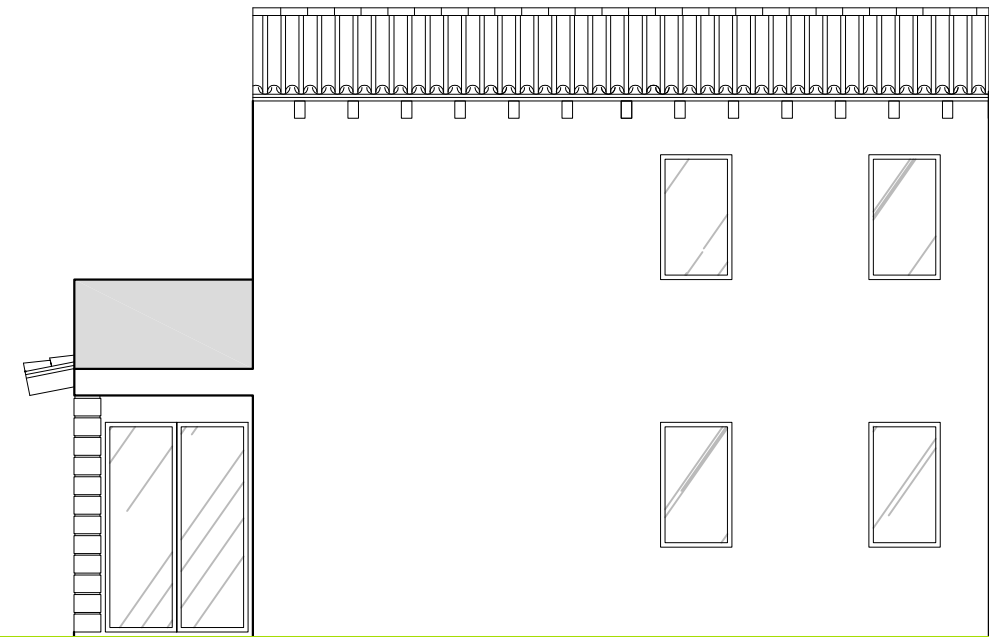
ALZADO LATERAL DERECHO
