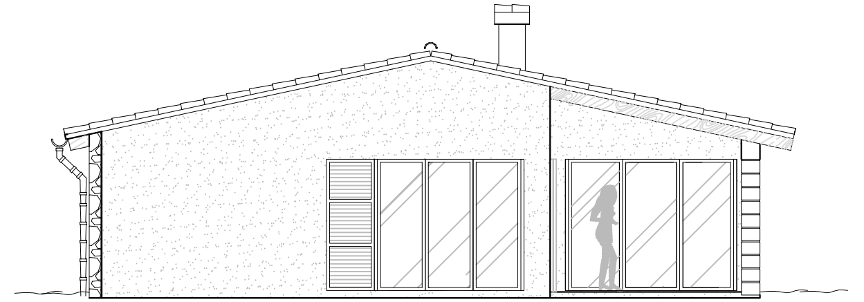
ALZADO LATERAL DERECHO
