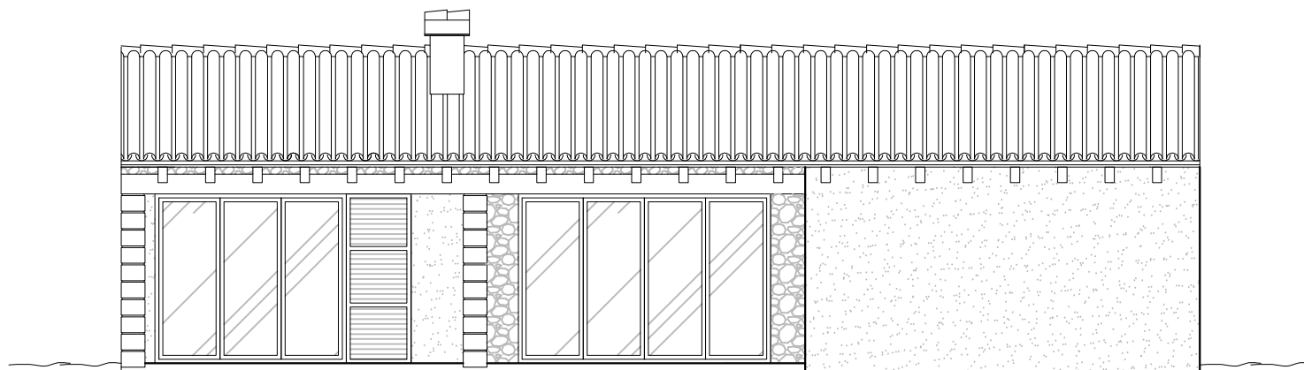
ALZADO POSTERIOR
