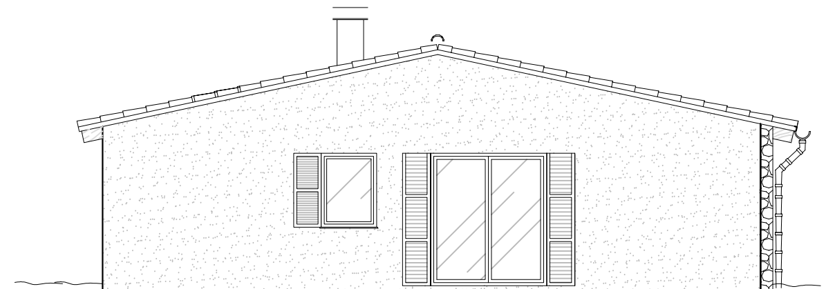
ALZADO LATERAL IZQUIERDO
